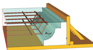
Coffrage sur plateau
