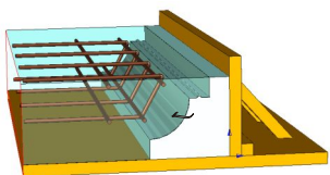
Coffrage sur plateau
