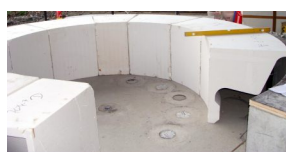
Goulottes rectilignes et cintrées Finlandaise - Wiesbaden - Saint Moritz
